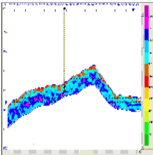
شکل ۹: مقطع امپدانس خط لرزه‌ای ۷۶۴۲۴ به شیوه بر مبنای مدل.
