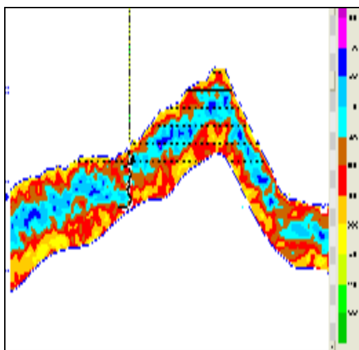
شکل ۱۰: مقطع امپدانس خط لرزه‌ای ۷۶۴۲۴ به شیوه خارهای پراکنده.
