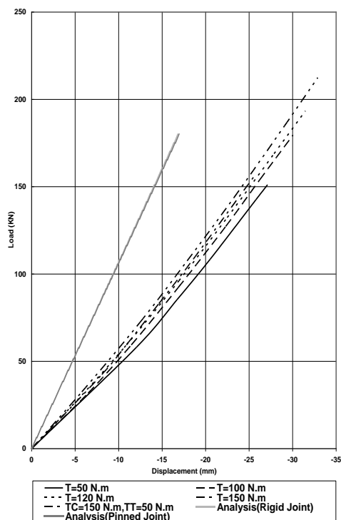
شکل ۷: نمودار نیرو تغییر مکان گره‌های گروه الف از مدل (۲) به روش تجربی و تحلیلی.
