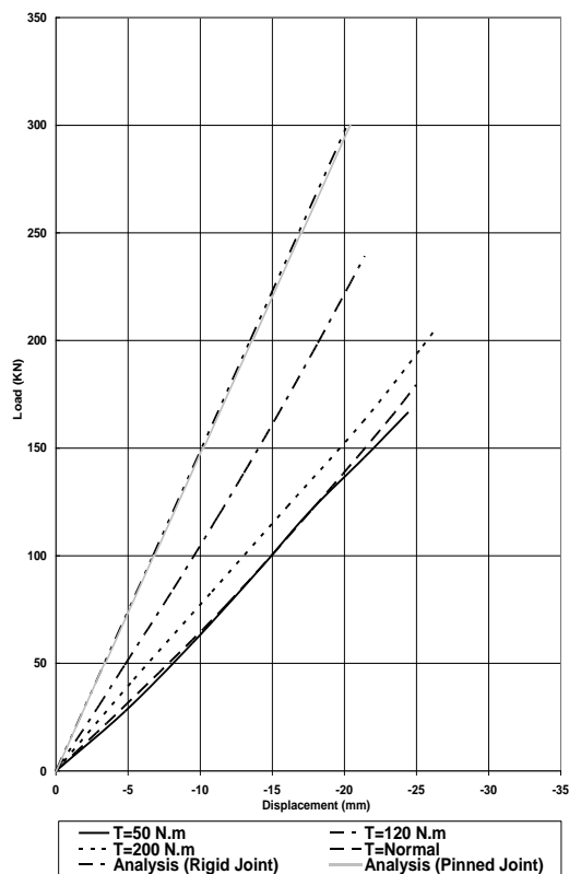
۴ : نمودار نیرو تغییر مکان گره‌های گروه الف از مدل (۱) به روش تجربی و تحلیلی.
