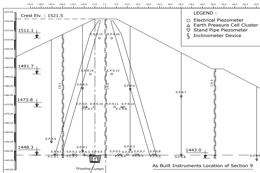
شکل ۱: آرایش ابزار در مقطع ۹-۹.
