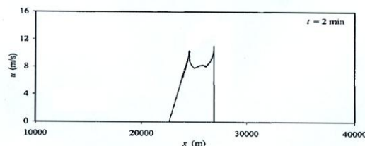
شکل ۱۹: پروفیل سرعت به دست آمده در مرجع [۱].
