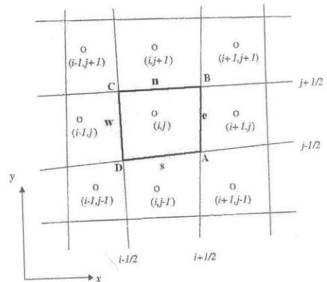
شکل ۱: سلولهای محاسباتی در مختصات x-y.
