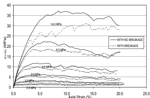
شکل ۶: تأثیر تنش همه‌جانبه بر روی تنش اختلافی
