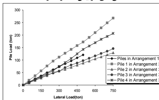
شکل ۱۲- مقایسه بار جانبی جذب شده به وسیله شمع‌های آرایش شماره ۱ و ۳
