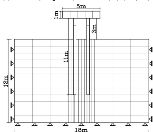
شکل ۴- ابعاد محیط و نوع تکیه گاه های مدل شده
